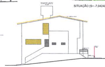
ELEVÇÃO SUL
