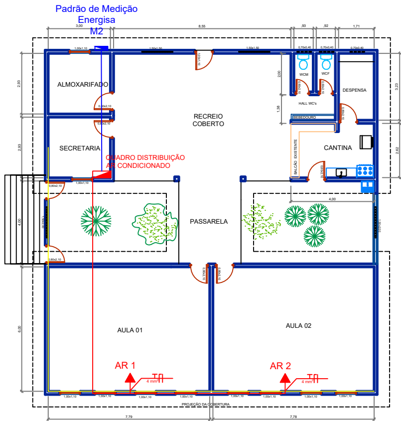
PLANTA BAIXA
