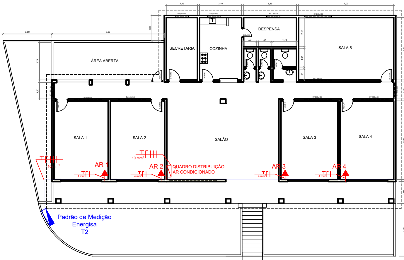
PLANTA BAIXA- 1:50
