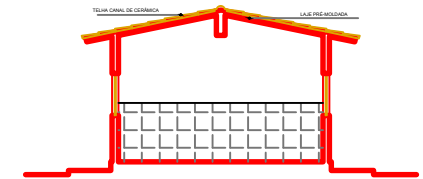
CORTE BB - 1: 50
