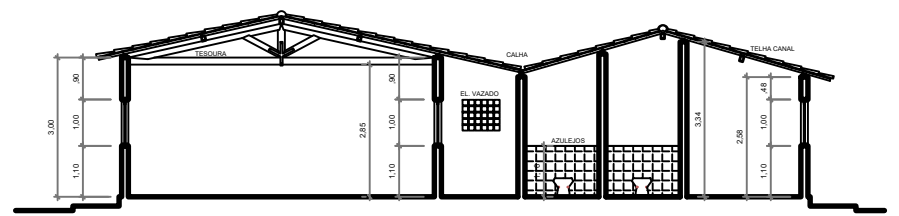
CORTE AA
