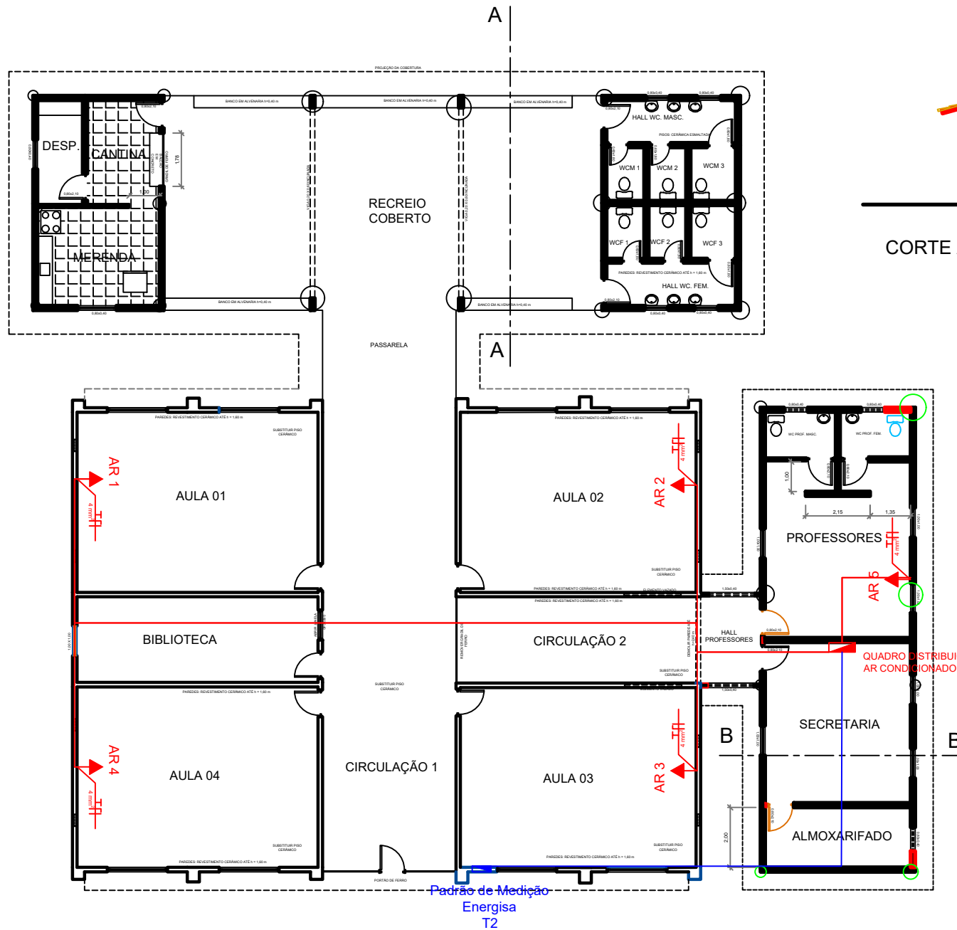
PLANTA BAIXA - 1: 50
