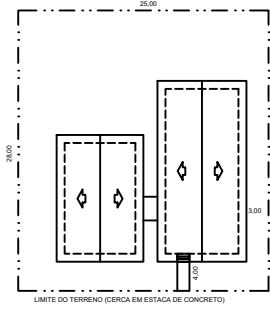
COBERTURA E LOCAÇÃO - 1:200
