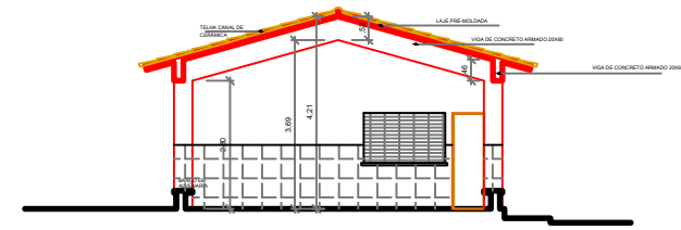
CORTE AA - 1: 50
