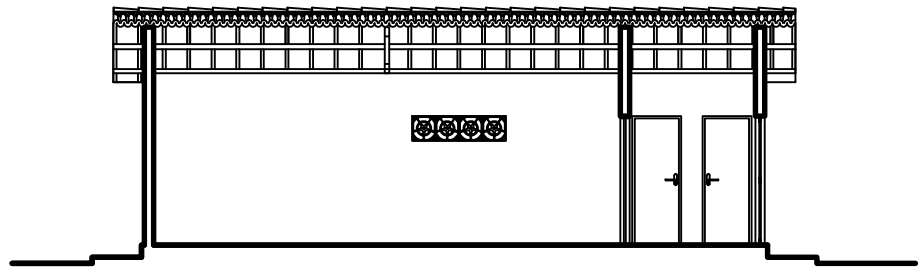
CORTE AA
