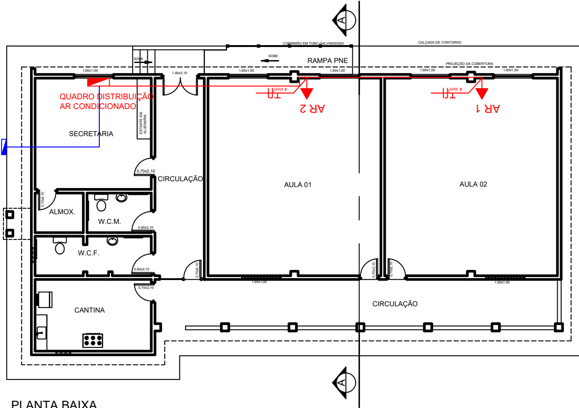
PLANTA BAIXA
