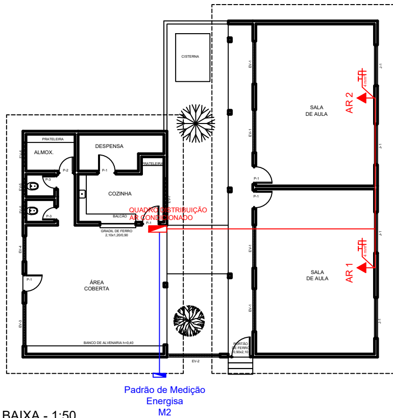
PLANTA BAIXA - 1:50
