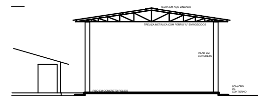
CORTE AA - ESC: 1:100
